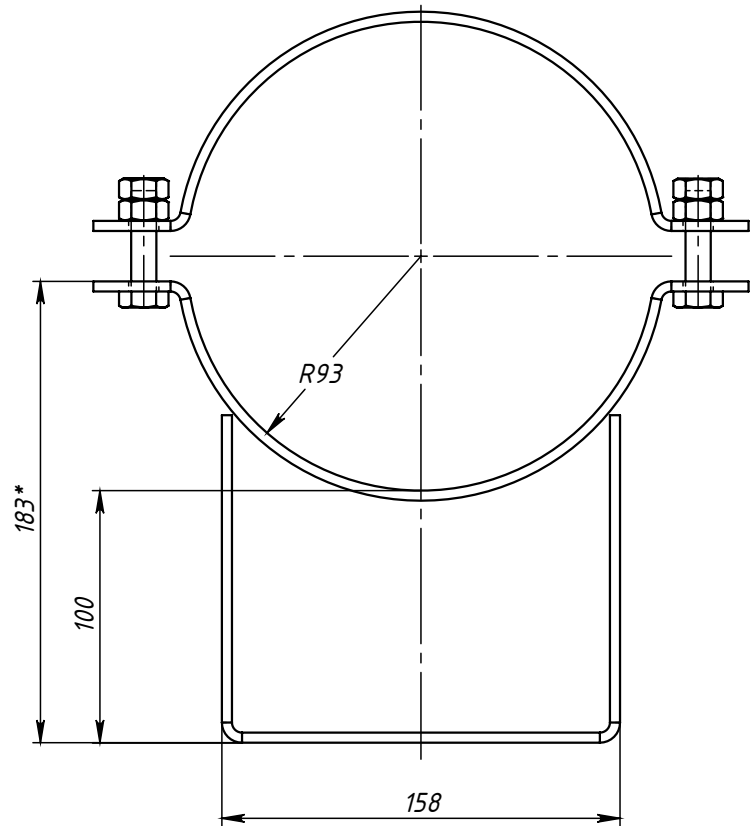
Поз.3 (Полухомут)
