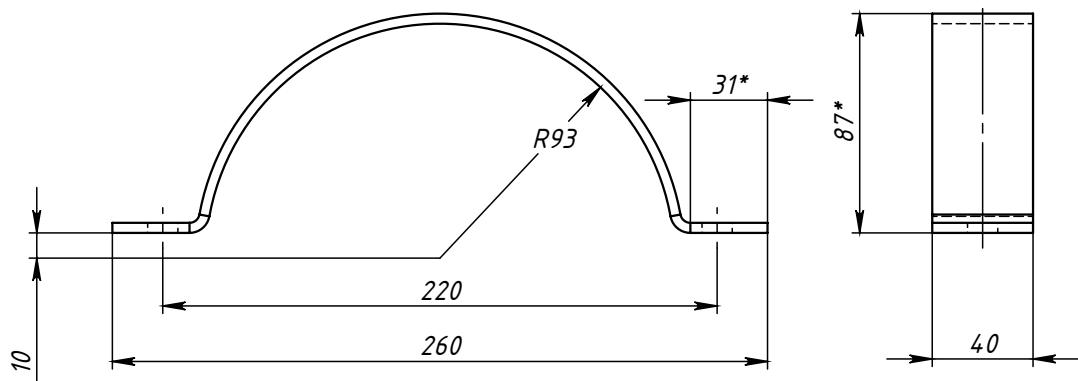
Поз.3 (Полухомут)
